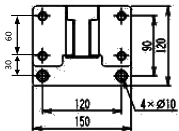
取付ベース寸法
